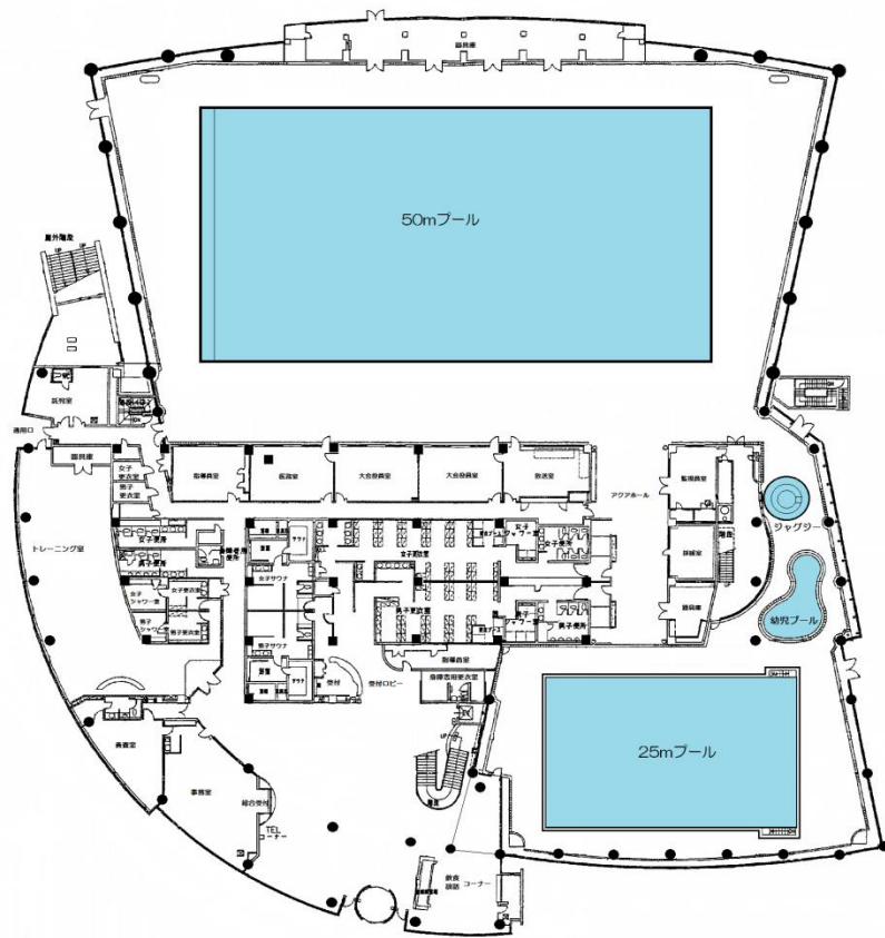
富山市民プール 1階平面図
